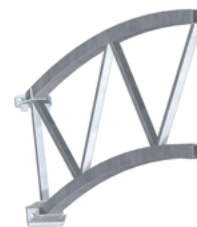
La poutre treillis permet d'élargir la portée en optimisant la matière. Le meilleur choix technique pour des portées supérieures à 15 m
